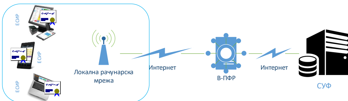
Слика: Један или више софтверских ЕСИР-а, инсталираних на личном рачунару, мобилном телефону или таблети, који се преко интернета повезују са софтверским виртуелним ПФР-ом
