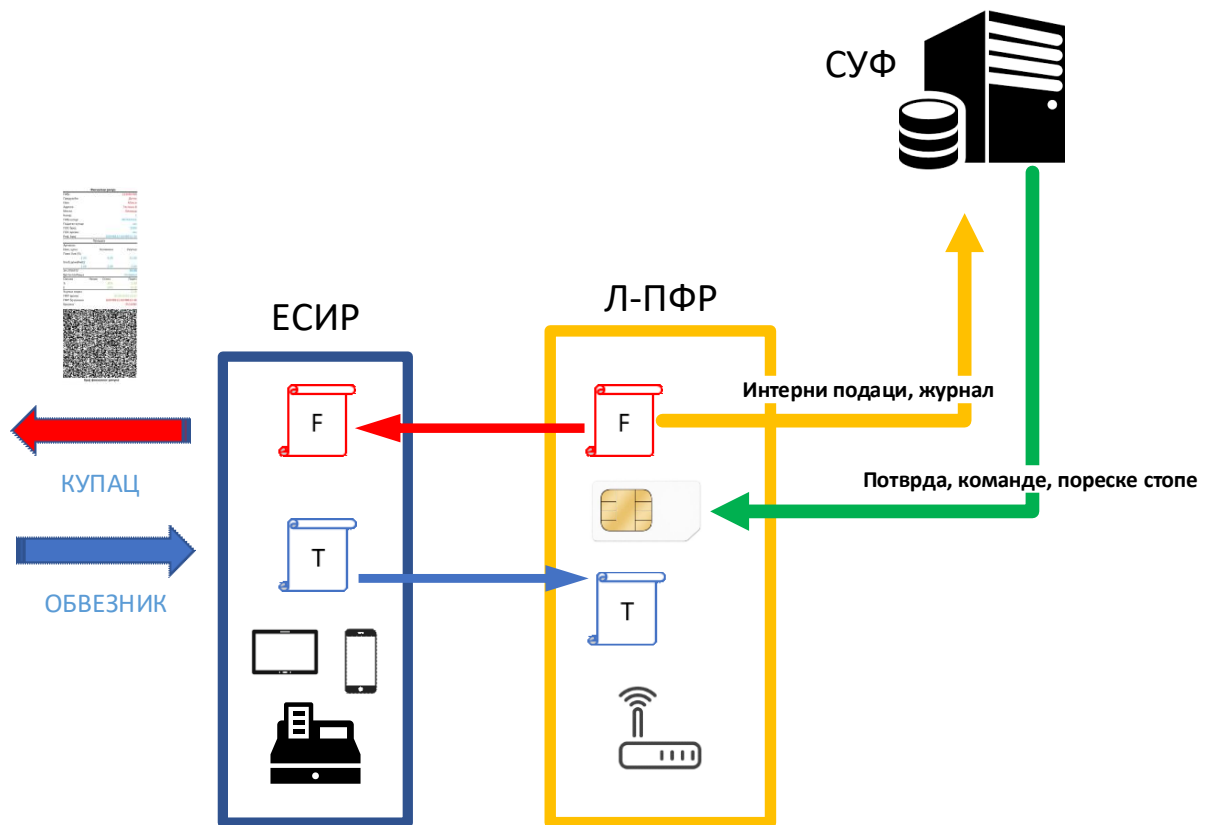
Слика: Интернет ишчитавање фискалих рачуна које генерише ЕФУ са Л-ПФР елементом и пренос података у СУФ помоћу било које доступне интернет везе
